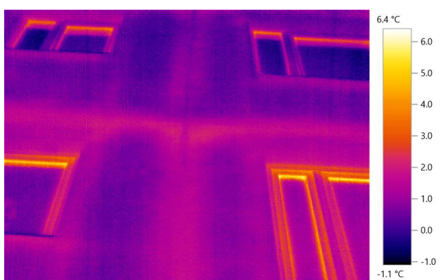
17.attēls. Ārsienas paneļu savienojuma vieta
