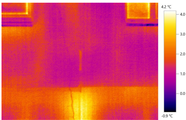
14.attēls. Paneļu šuves
