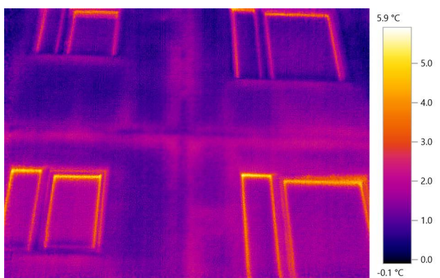
18.attēls. Ārsienas paneļu savienojuma vieta
