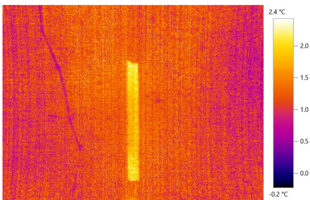
15.attēls. Paneļu šuve
