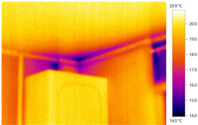
19.attēls. Temperatūras pazemināšanās ēkas stūrī
