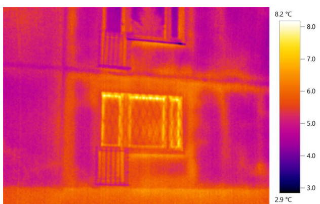
8.attēls. Ēkas ziemeļu fasāde, paaugstināta virsmas temperatūra uz loga rāmja, paneļu šuvju vietās
