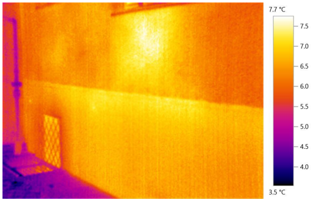
13.attēls. Ēkas austrumu fasāde
