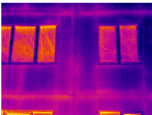
5.attēls. Lokāla temperatūras paaugstināšanās paneļu šuvju vietās
