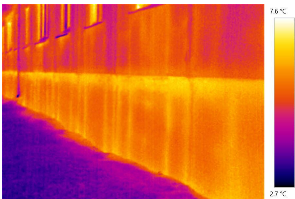
24.attēls. Ēkas austrumu fasādes cokols
