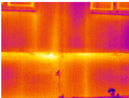
8.attēls. Virsmas temperatūras paaugstināšanās ārsienas/cokola mezglā
