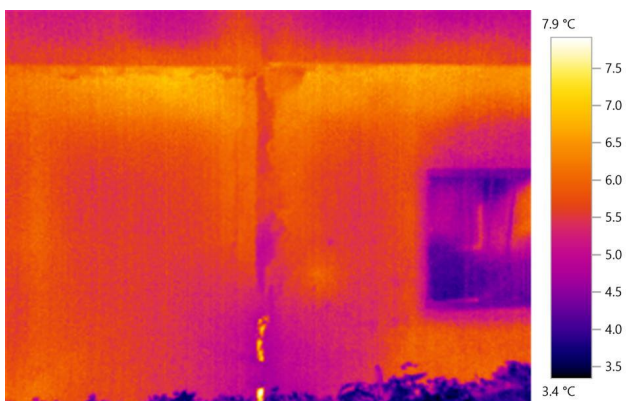
21.attēls. Cokola paneļu savienojums
