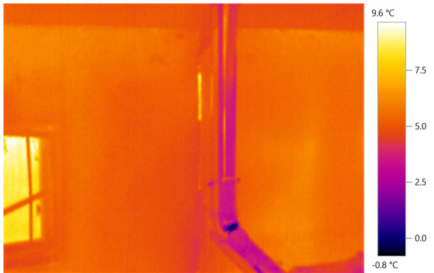
22.attēls. Cokola paneļu savienojums
