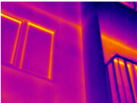
2.attēls. Balkona termiskais tilts, siltuma zudumi caur loga rāmi
