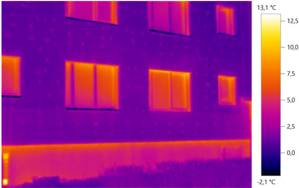
1. att. Ēkas fasāde (siltināta) un cokols (nesiltināts)
