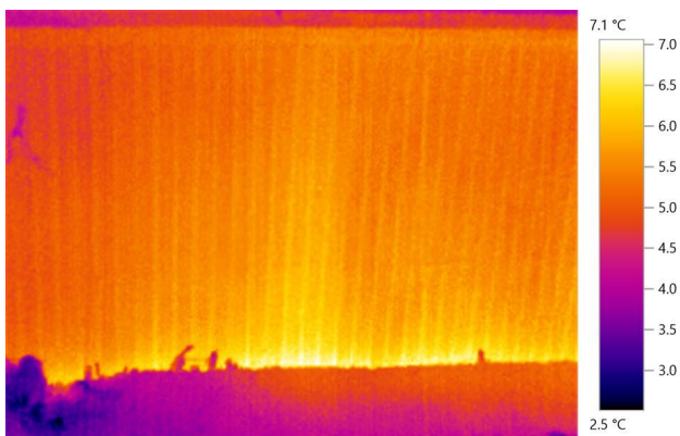
5.attēls. Siltuma zudumi caur ēka cokolu
