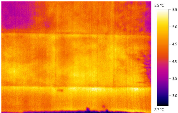
4.attēls. Ēkas rietumu fasāde
