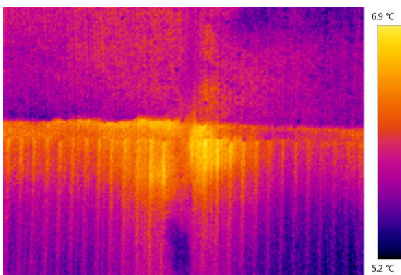
21.attēls. Paneļu savienojuma vieta
